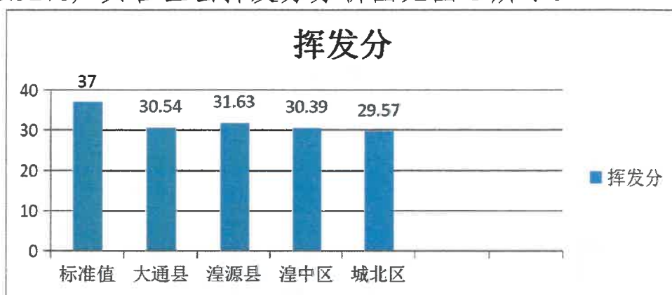
图 1 挥发分分析图
